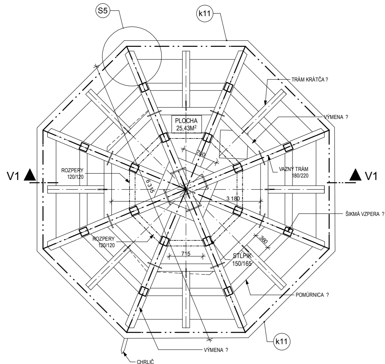
PÔDORYS KONŠTRUKCIE KROVU STRECHY VEŽE V ÚROVNI NAD VÁZNÝMI TRÁMAMI
